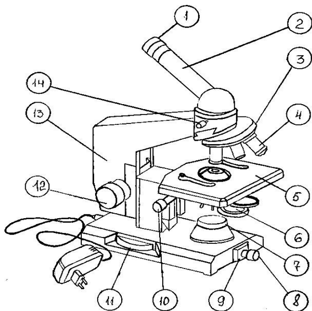
Рисунок 1. Микроскоп МБР-1
